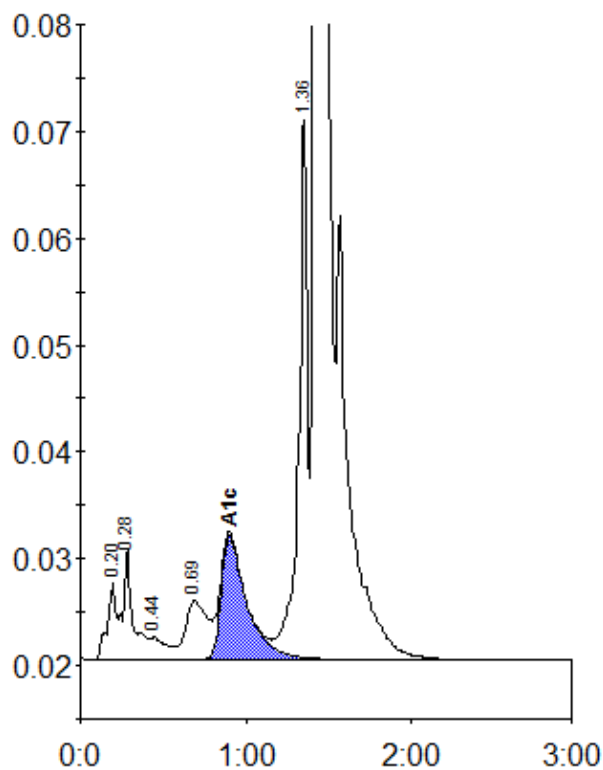
Peak table - ID: 10433297
